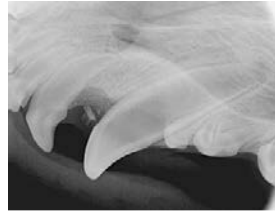
Kuva 3.c: Vas. yläkulmahammas.
