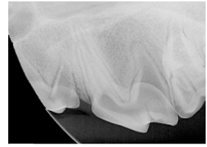
Kuva 3.d: Vas. ylä-P4-M2.
