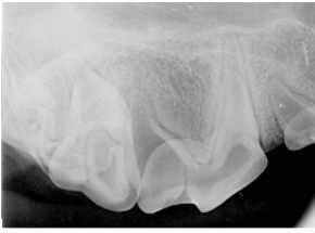
Kuva 3.a: Oik. ylä-P4-M2.
