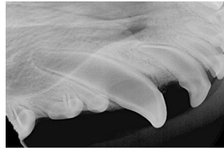
Kuva 3.b: Oik.yläkulmahammas.
